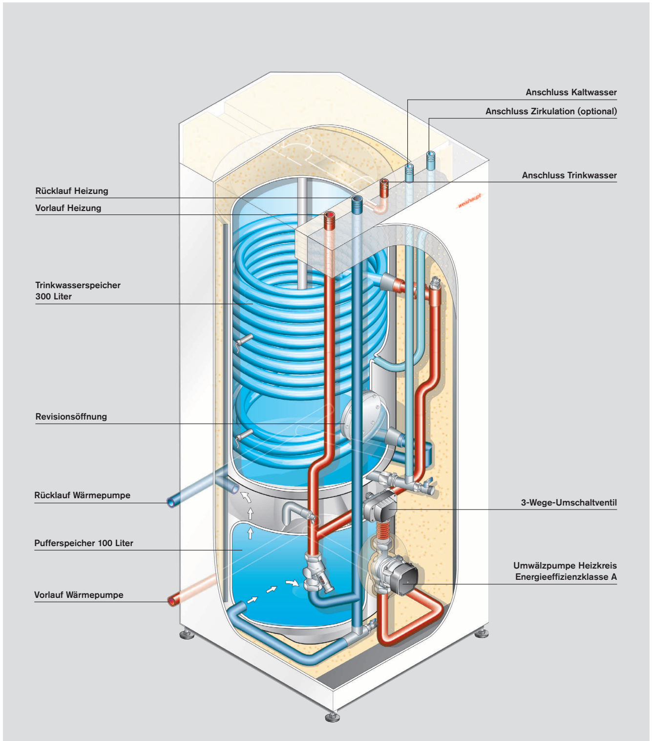
Weishaupt Kombispeicher WKS 300 / 100 LE / Unit-E / Bloc / C für Biblock-Wärmepumpen
