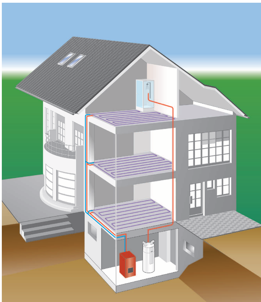
Trinkwasser-Wärmepumpe
